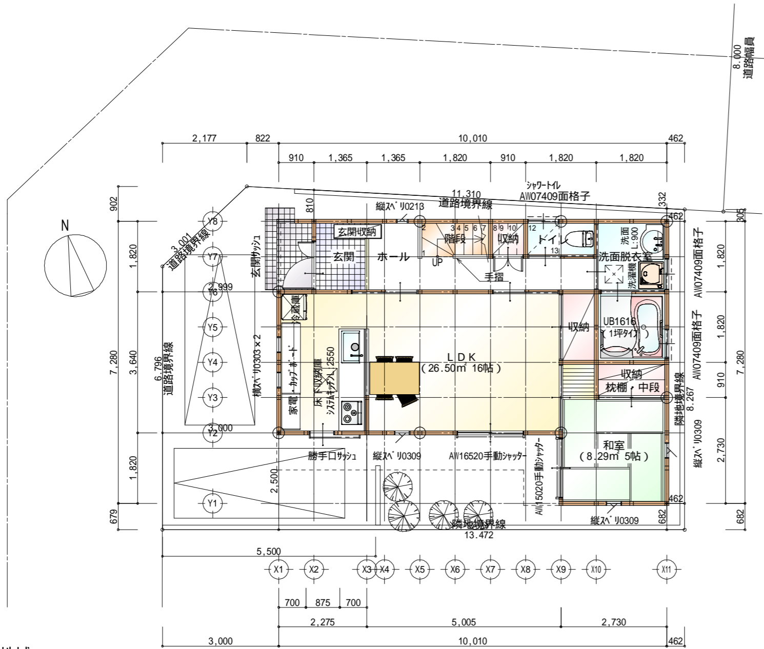
配置図 S:1/100
