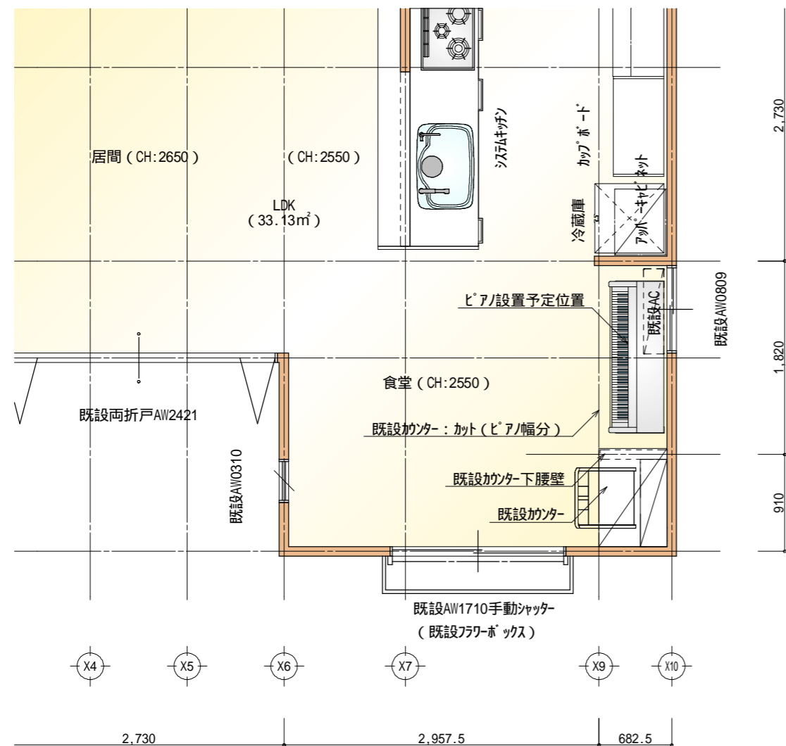
1階 平面図 S: 1/50
