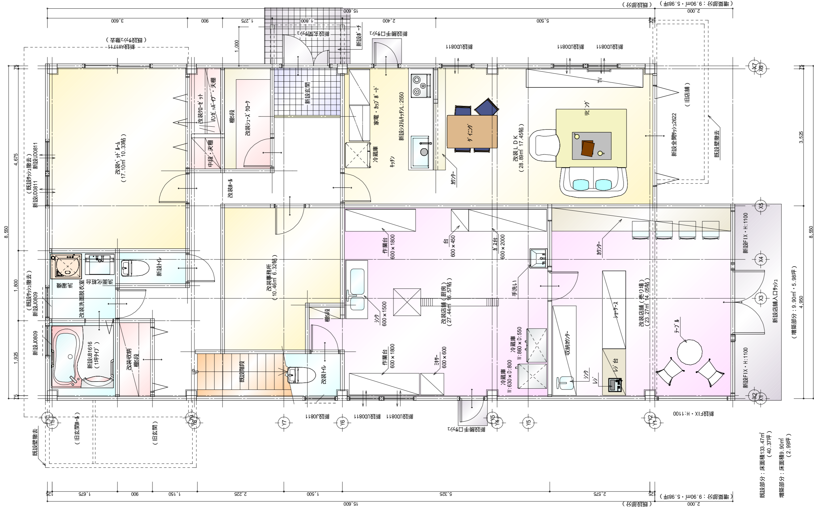
1階平面図 S:1/60
